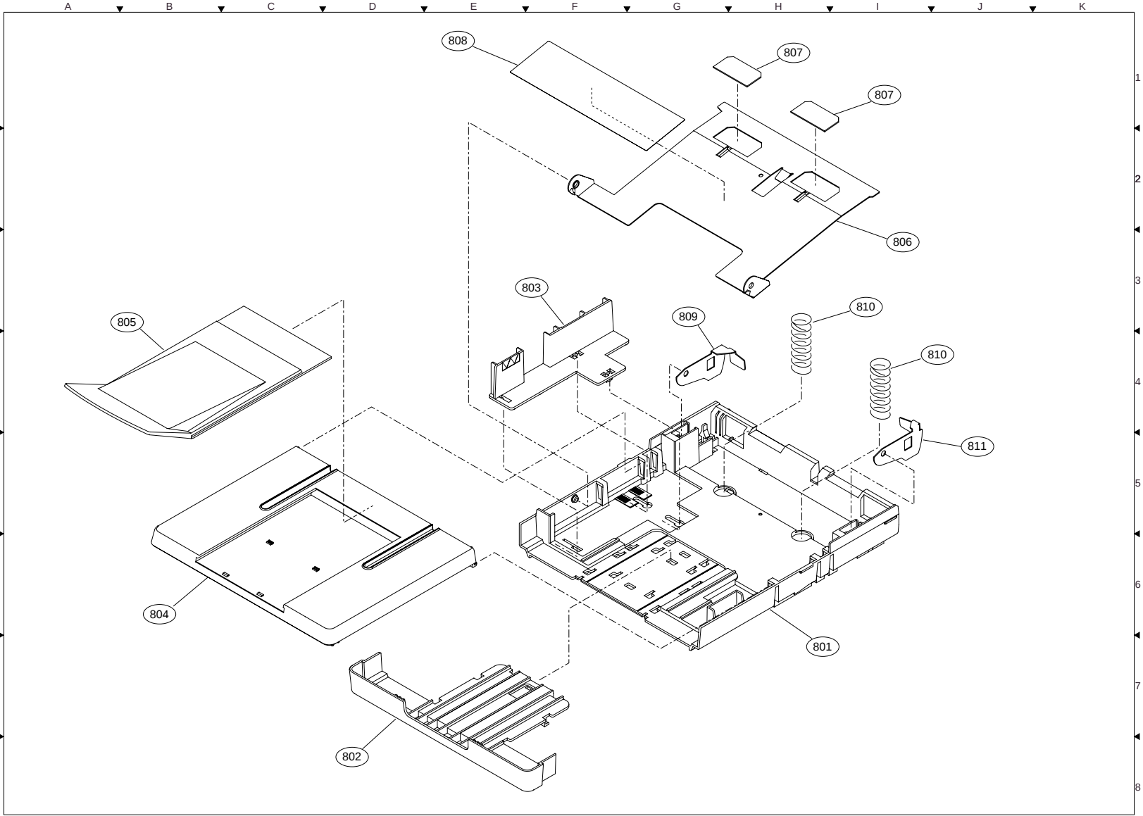
FIG. 8 CASSETTE
