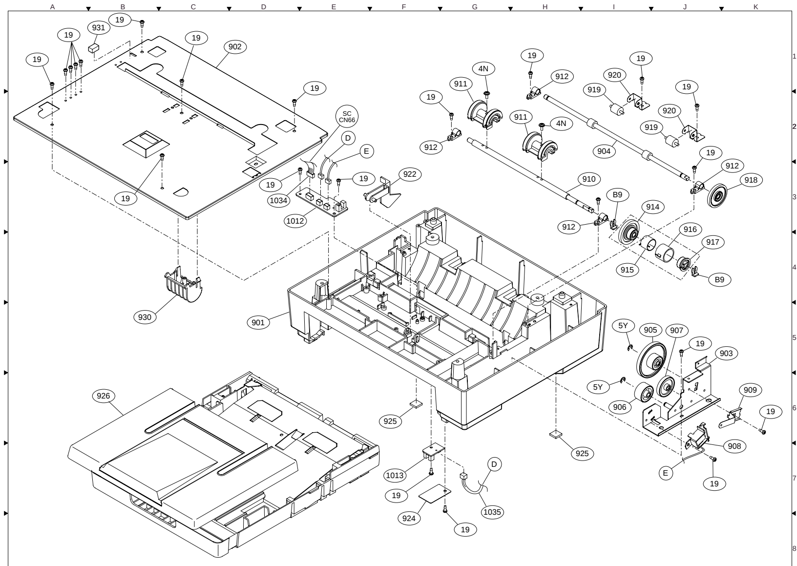
FIG. 9 OPTION CASSETTE
